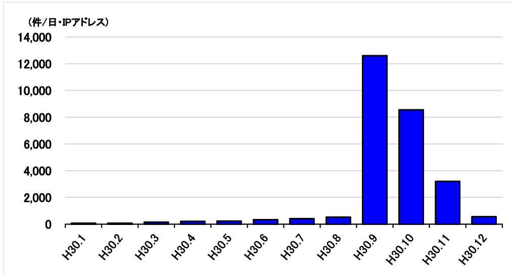
【図表4 宛先ポート80/TCPに対するアクセス件数の推移】
